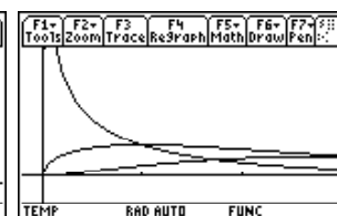
図 23: \chi^2 分布
